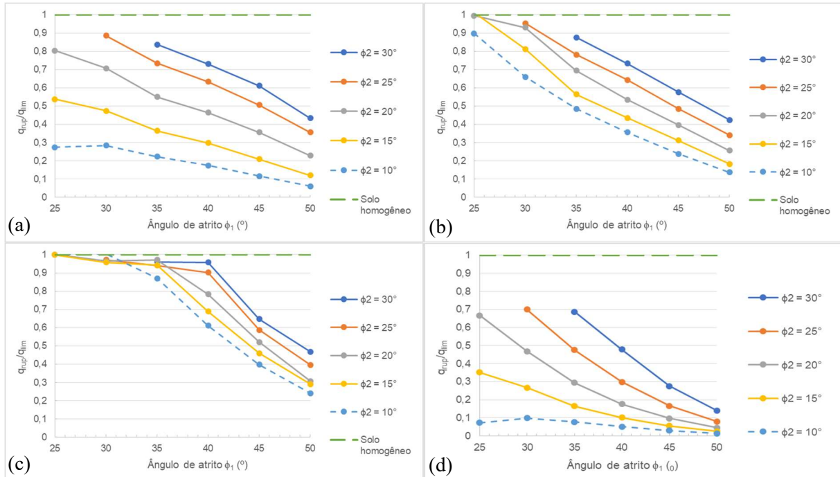
Figura 4. Redução da capacidade de carga. (a) z_i/B = 0,50 , h_0 = 0,10\text{ cm} ; (b) z_i/B = 1,00 , h_0 = 10\text{ cm} ; (c) z_i/B = 1,50 , h_0 = 10\text{ cm} ; (d) z_i/B = 0,50 , h_0 = 30\text{ cm} .
