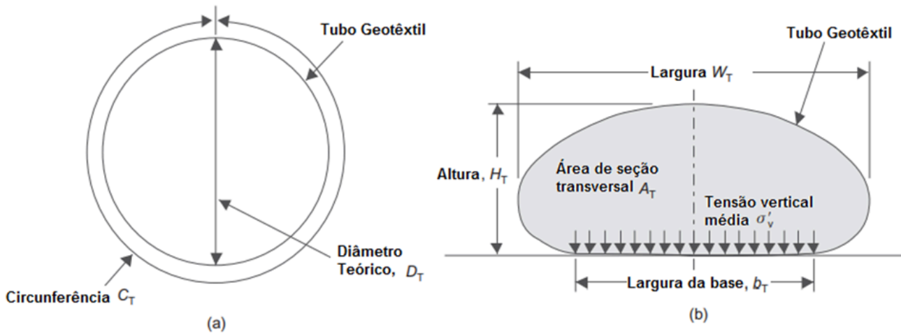
Figura 6. Parâmetros fundamentais do tubo geotêxtil (a); parâmetros de engenharia importantes para tubos geotêxteis cheios (b) (traduzido e adaptado de LAWSON, 2008).
