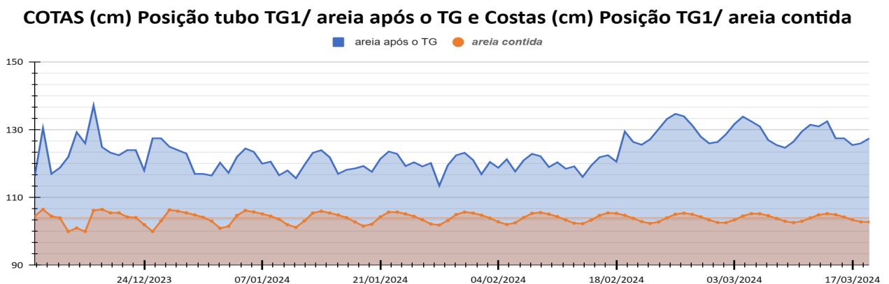
Figura 8. Variação das cotas de areia antes e depois da contenção com os tubos de geotêxtil.
