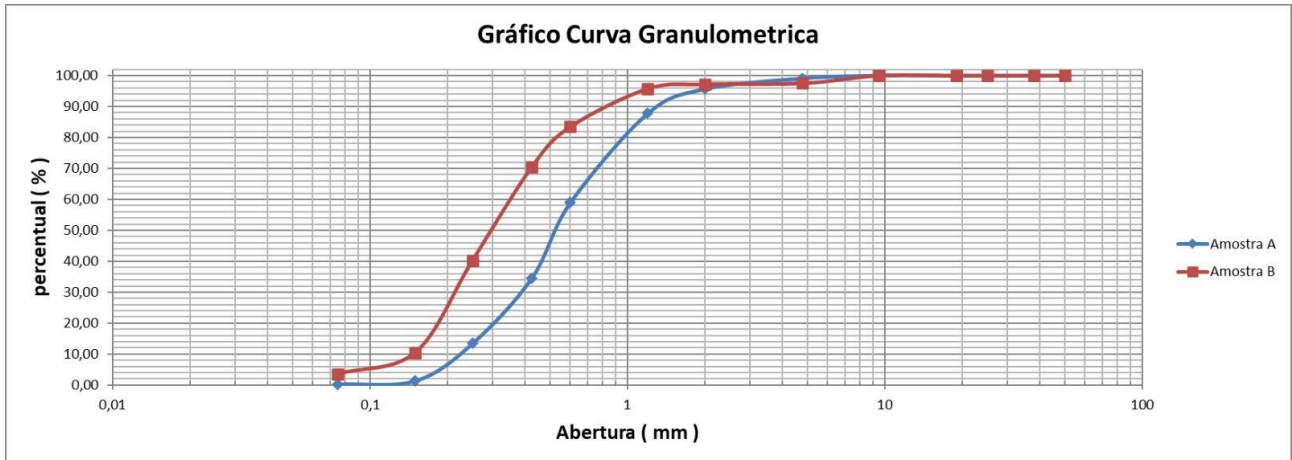
Figura 4. Gráfico de Curva Granulométrica.
