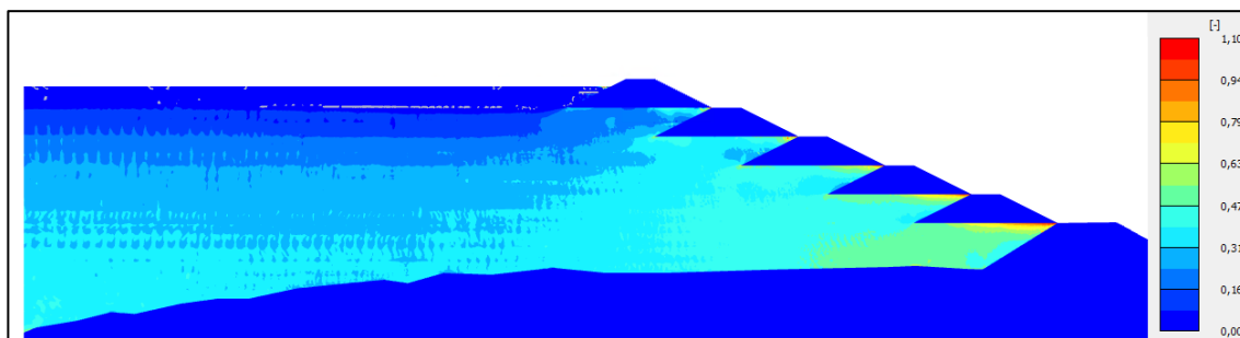
Figura 6. Razão de Resistência Normalizada ( N/M_{\theta} ) – Pré obra de reforço e escavação – Simulação apenas com Norsand .
