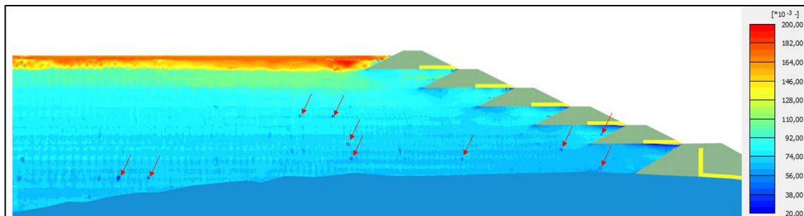
Figura 4. Parâmetro de Estado – Pré obra de reforço e escavação – Simulação apenas com Norsand – Destaque em vermelho para regiões pontuais com valores discrepantes de \Psi .
