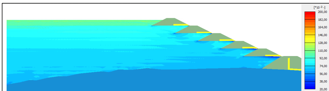
Figura 5. Parâmetro de Estado – Pré obra de reforço e escavação – Simulação alternando Norsand e HSM.
