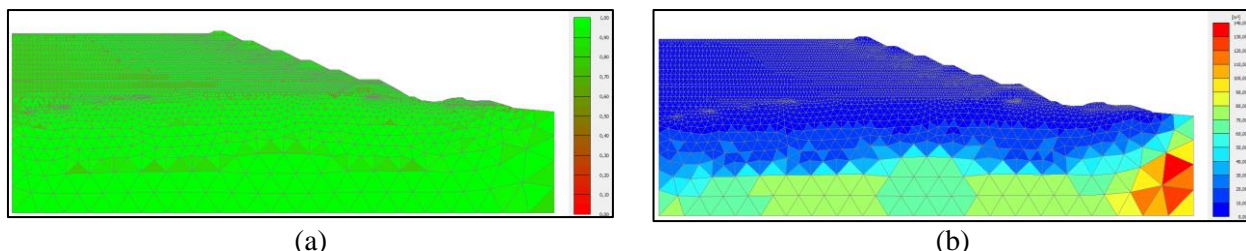
Figura 2. (a) Qualidade da malha de elementos finitos; (b) Área dos elementos da malha.
