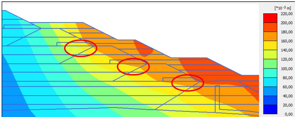
Figura 3. Deslocamento Total – Pós obra de reforço e escavação – Simulação alternando Norsand e HSM – Destaque para regiões no qual foram identificados maiores valores de deslocamento e deformação no rejeito.
