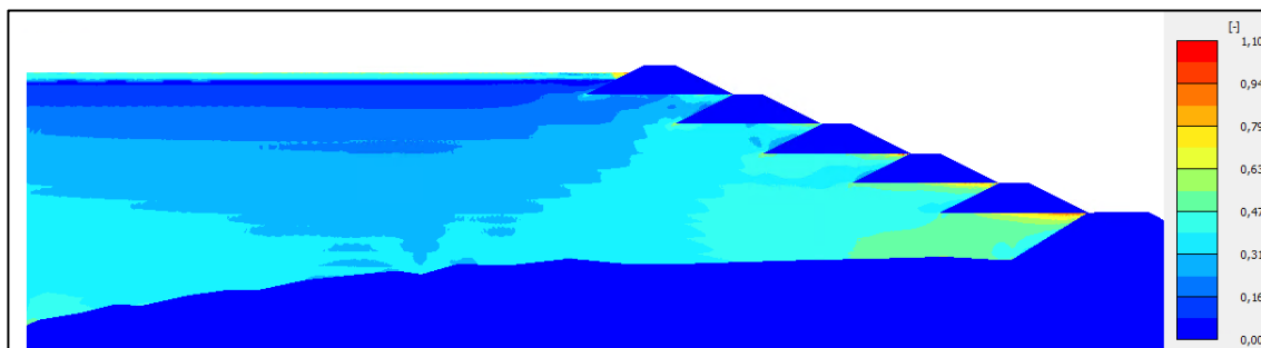
Figura 7. Razão de Resistência Normalizada ( N/M_{\theta} ) – Pré obra de reforço e escavação – Simulação alternando Norsand e HSM.
