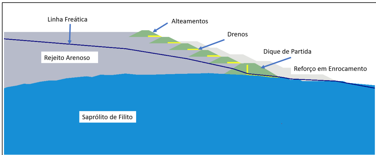
Figura 1. Seção Geológico-Geotécnica e Linha Freática utilizada como para o estudo.
