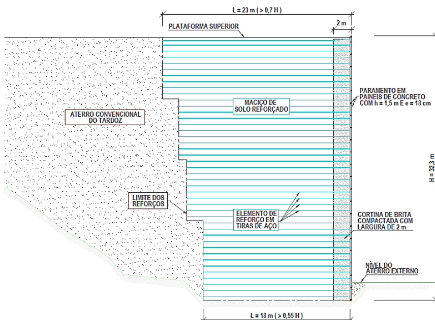
Figura 6 – Seção transversal típica da estrutura considerada, com a aplicação da cortina de brita compactada no tardo do paramento.
