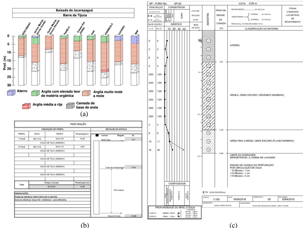
Figura 3. (a) Perfis típicos da Baixada de Jacarepaguá - (adaptado de BARONI, 2016 apud RICCIO et al. , 2013); (b) boletim de cravação da estaca (Tsuchiya, 2021); (c) Boletim de sondagem (Tsuchiya, 2021)
