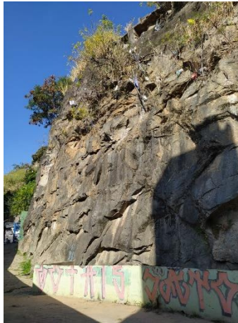
Figura 1. Vista do talude.
