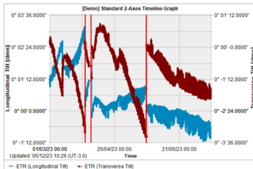
Figura 5 – Gráficos de Longitudinal and Transverse Tilt (Nível transversal e longitudinal) impactados pelo desnivelamento do equipamento indicado através das 3 linhas verticais em vermelho na figura. (Fonte: Vale & Hexagon)
