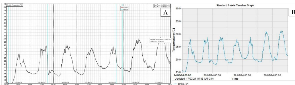
Figura 8 – Gráficos de Temperatura da estação meteorológica acoplada ao radar IBIS-FM (Figura A) e do sensor de temperatura e pressão da estação total robótica (Figura B). (Fonte: Vale & Hexagon)
