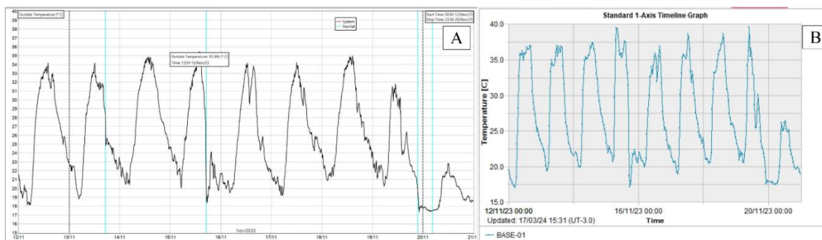
Figura 7 – Gráficos de Temperatura da estação meteorológica acoplada ao radar IBIS-FM (Figura A) e do sensor de temperatura e pressão da estação total robótica (Figura B). (Fonte: Vale & Hexagon)
