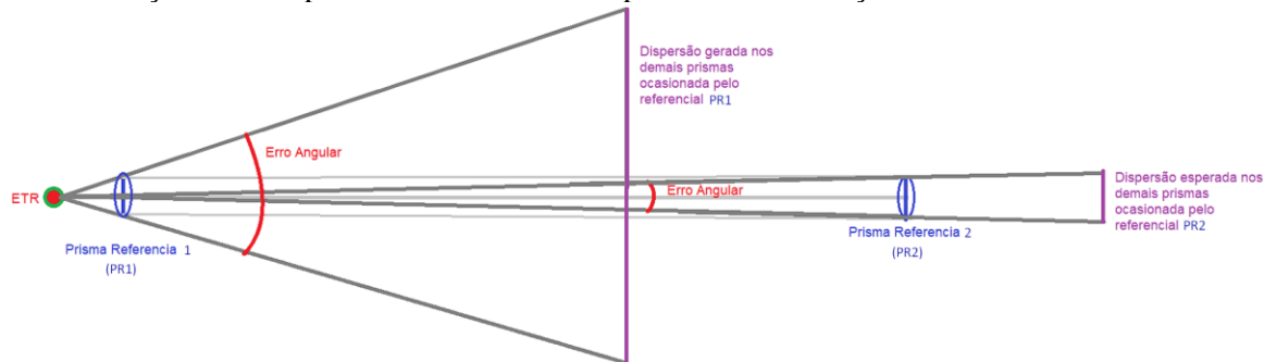
Figura 2 – Representação gráfica da influência da distância entre a estação total e os prismas alvo e referenciais nos dados angulares horizontais. (Fonte: Elaboração Própria.)
