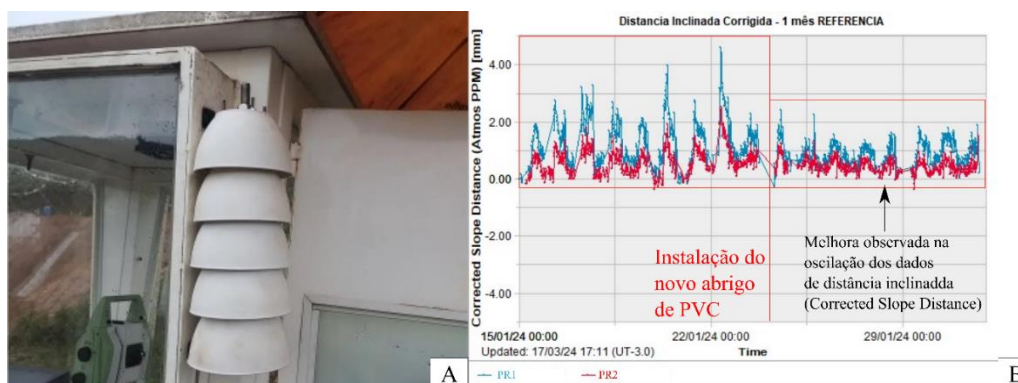
Figura 9 – Exemplo do abrigo feito de PVC para o sensor de temperatura e pressão e gráficos de Corrected Slope Distance (Distância Inclinada Corrigida) para os prismas referenciais da estrutura monitorada. (Fonte: Vale & Hexagon)
