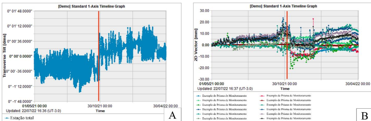
Figura 4 – Gráficos de Transverse Tilt (Nível transversal), Figura A, e Vector 2D de prismas de monitoramento de um sistema de monitorado por uma TM50, Figura B, impactados pelo desnivelamento do equipamento indicado através de uma linha vertical em vermelho na figura. (Fonte: Vale & Hexagon)
