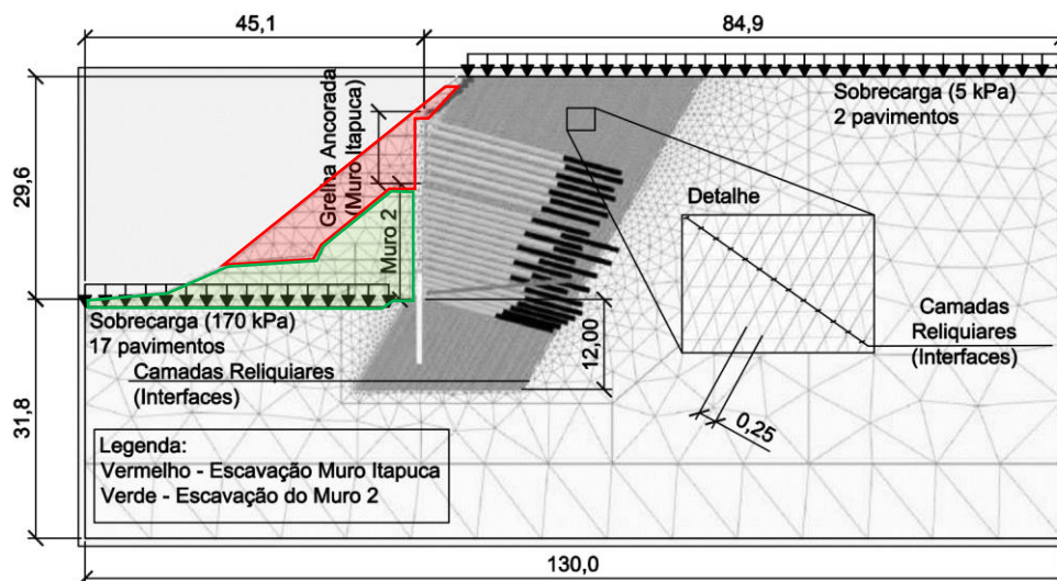
Figura 4 – Modelo de elementos finitos validado (Moura et. al. , 2023). Dimensões em metros.
