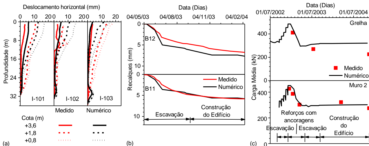
Figura 5 - Dados de instrumentação validados: (a) inclinômetros, (b) marcos superficiais à montante e (c) cargas nas ancoragens (Moura et. al , 2023).
