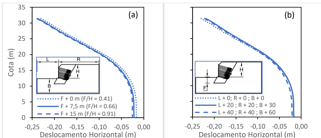
Figura 3 - Análise de sensibilidade: (a) condições de contorno (b) fundação das camadas reliquias fracas.
