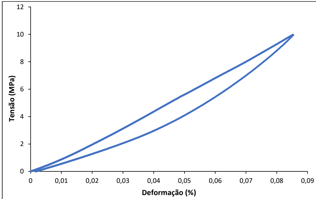
Figura 6. Curva tensão x deformação
