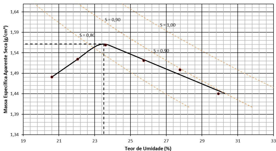
Figura 2: Curva de compactação do solo residual de gabro.
