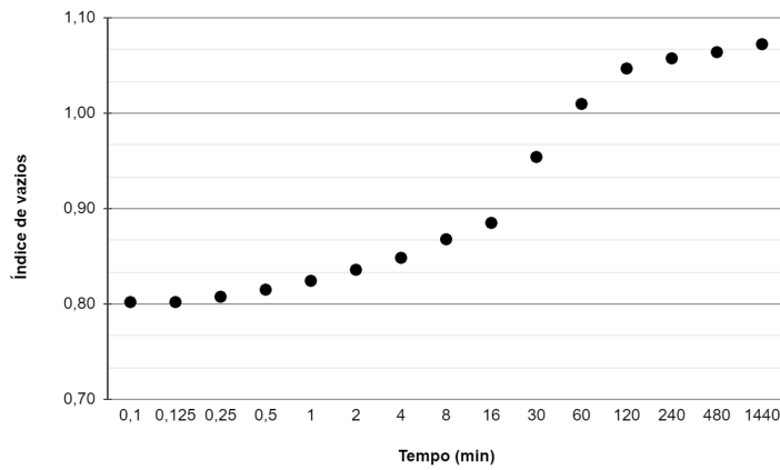
Figura 4. Ensaio de expansão unidimensional com carga de 10kPa.
