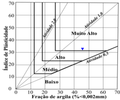
Figura 3: Diagrama de Van der Merwe com a indicação (triângulo azul) do potencial de expansão do solo em estudo.
