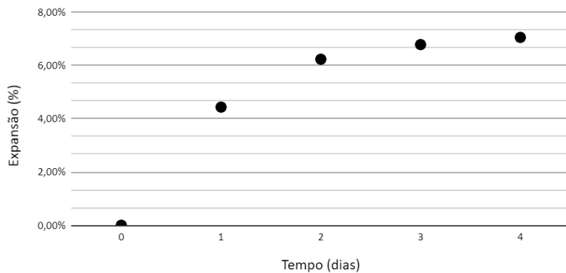
Figura 5. Curva de expansão do ensaio CBR.
