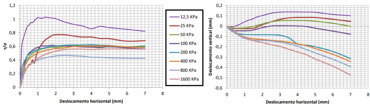
Figura 4 – Resultados do ensaio de cisalhamento direto para compactidade medianamente compacta da areia da praia de Cavaleiros - adaptado de Pinheiro (2018).
