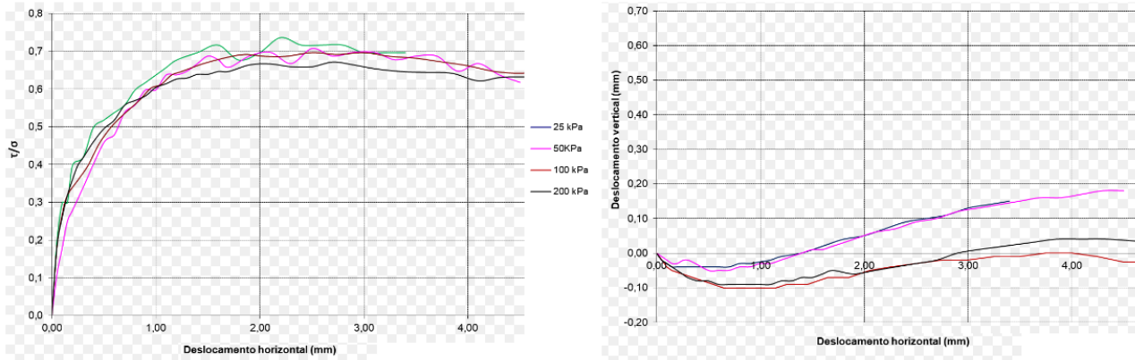
Figura 7 – Resultados do ensaio de cisalhamento direto para compactidade medianamente compacta da areia de Hokksund - adaptado de Marques e Oliveira (2009).
