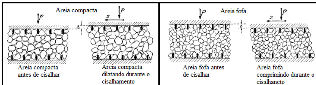
Figura 1 – Comportamento de areia – Adaptado de Casagrande (1936).
