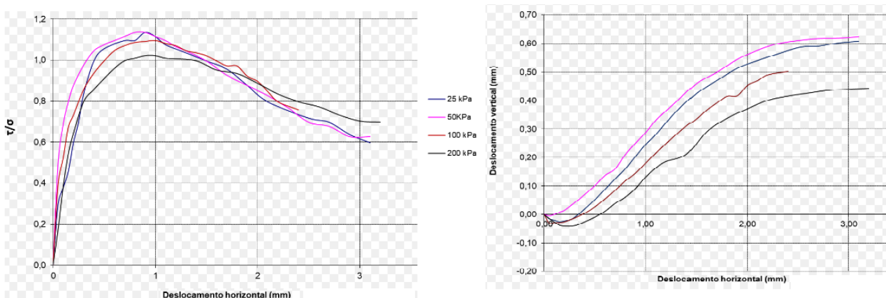
Figura 9 – Resultados do ensaio de cisalhamento direto para compactidade compacta da areia de Hokksund - adaptado de Marques e Oliveira (2009).
