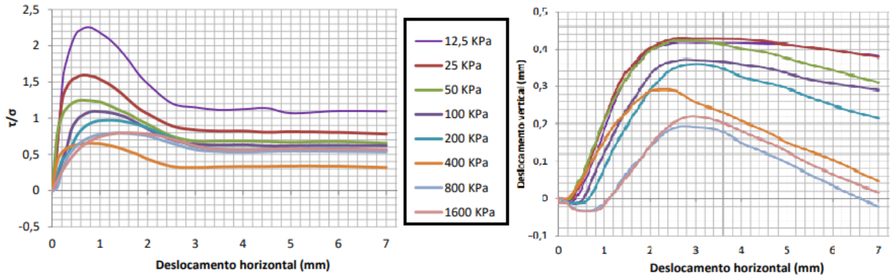
Figura 5 – Resultados do ensaio de cisalhamento direto para compactidade compacta da areia da praia de Cavaleiros - adaptado de Pinheiro (2018).
