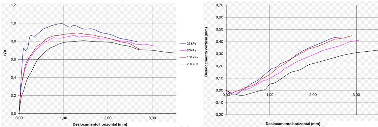
Figura 8 – Resultados do ensaio de cisalhamento direto para compactidade medianamente compacta da areia de Hokksund - adaptado de Marques e Oliveira (2009).
