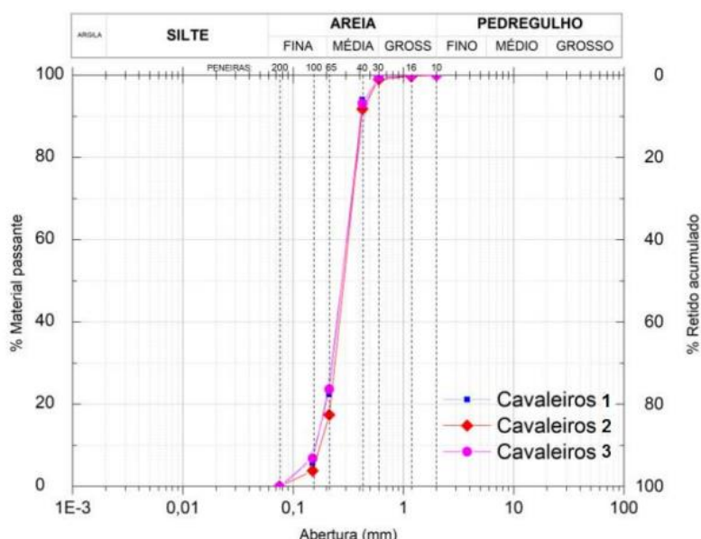
Figura 2 – Curvas granulométricas da areia da praia de Cavaleiros – Adaptado de Pinheiro (2018).
