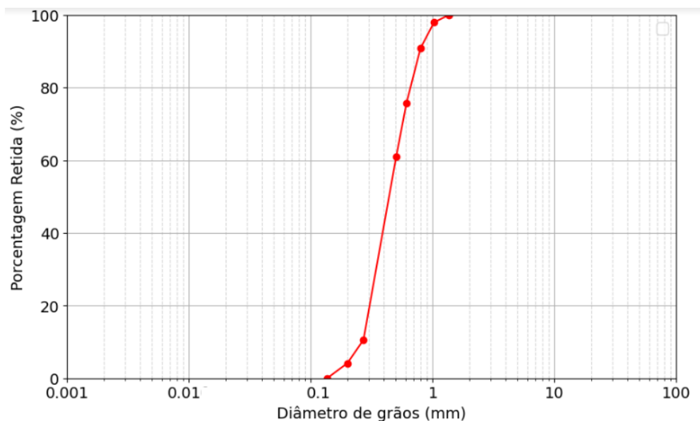
Figura 6 – Curva granulométrica da areia de Hokksund na Noruega – Adaptado de Parkin e Lunne (1982)
