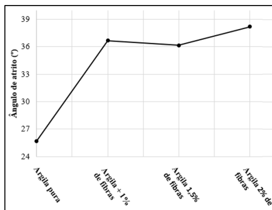
Figura 7. Comparativo de valores de ângulo de atrito.
