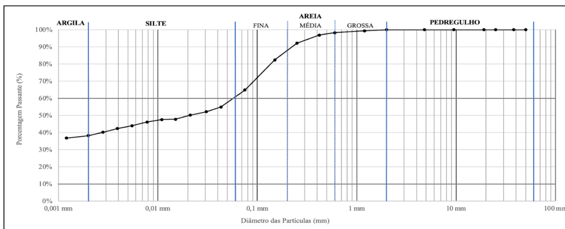
Figura 2. Curva granulométrica do solo.
