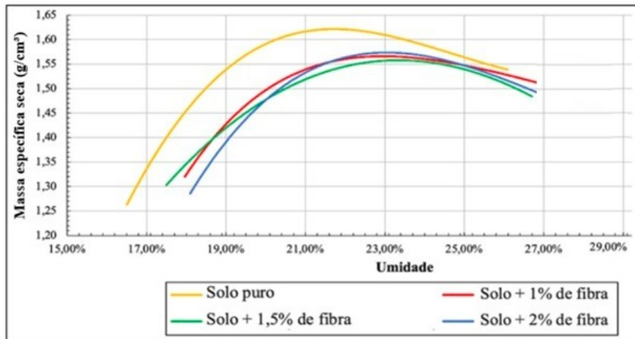
Figura 4. Curvas de compactação das amostras.
