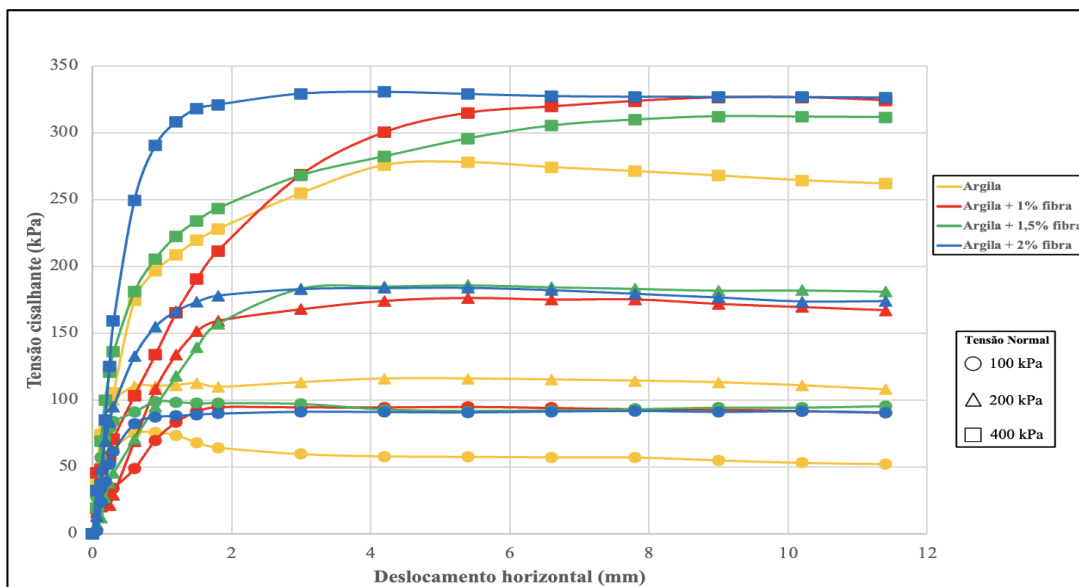
Figura 5. Tensão cisalhante vs deslocamento horizontal.
