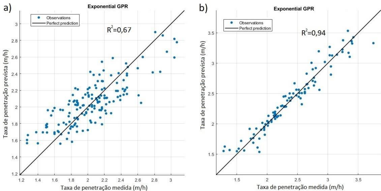
Figura 3. Diagrama de distribuição da taxa de penetração medida e prevista para o a) Banco de dados 1 e o b) Banco de dados 2.
