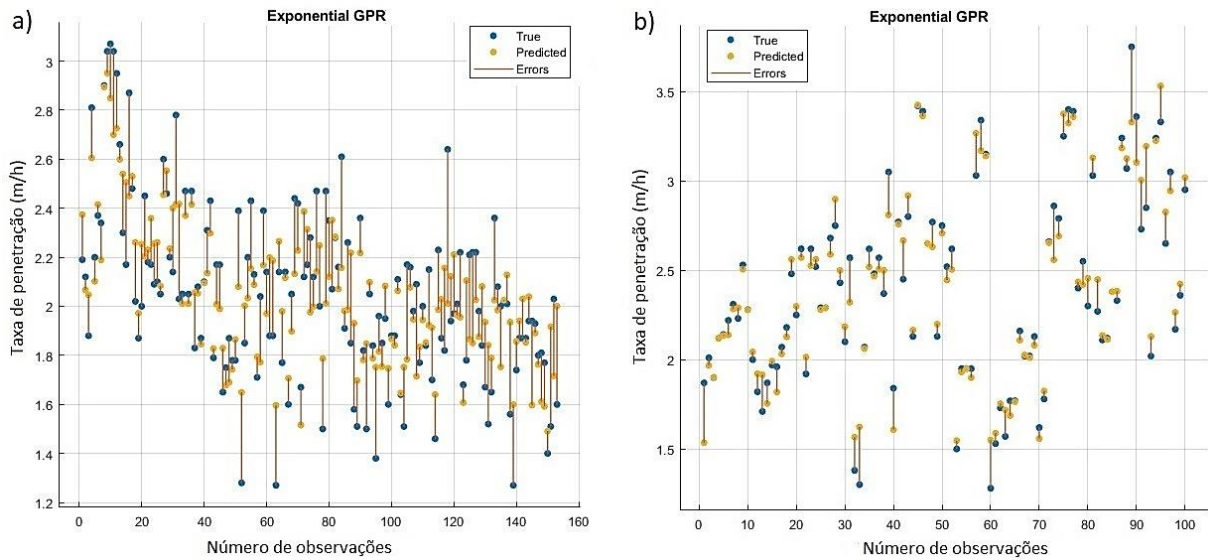
Figura 2. Diagrama de ajuste da Taxa de Penetração medida e prevista para o a) Banco de dados 1 e o b) Banco de dados 2.
