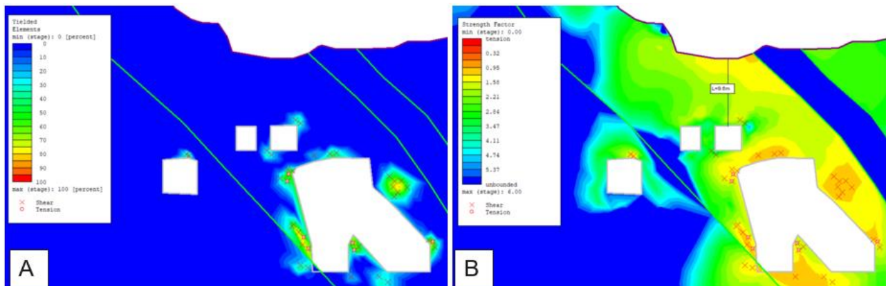
Figura 7: Exemplos de análises numéricas bidimensionais para dimensionamento do crown pillar ideal. A) avaliação em termos de zona de plastificação – yielded elements e B) avaliação em termos de strength factor .
