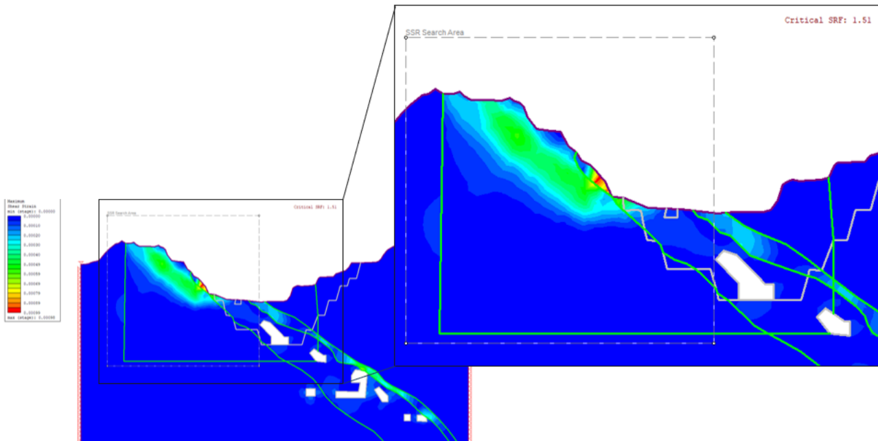
Figura 6: Condição de deformação máxima de cisalhamento, indicando valores de SRF iguais a 1.51. Para esse cenário é possível observar que não há interferência das escavações com
