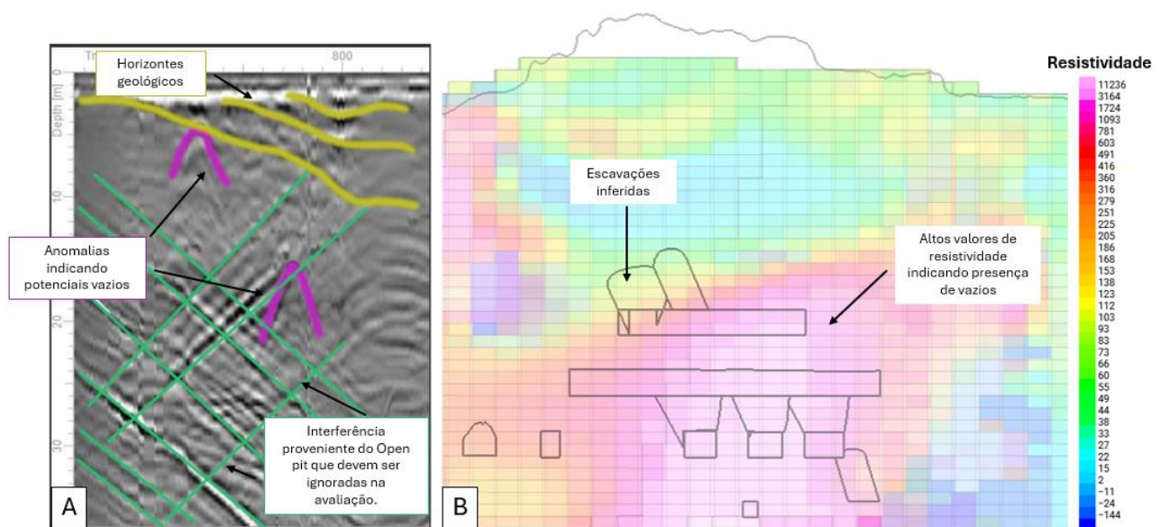
Figura 5: A) Interpretação dos resultados geofísicos obtidos através do GPR, estando em rosa a interpretação de potenciais vazios. B) Seção com valores de resistividade, sendo os valores baixos interpretados como solos argilosos e/ou rochas alteradas, valores médios interpretados como rocha e valores acima de 10.000 tratados como anomalias, podendo as mesmas serem indicativas de vazios.
