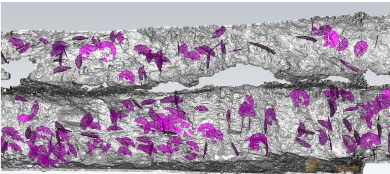
Figura 4: Discos estruturais obtidos por meio de aerofotogrametria e mapeamentos em campo.
