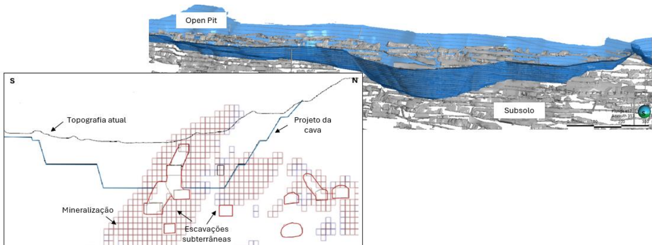
Figura 3: Croqui esquemático indicando interação entre Open Pit e subsolo.
