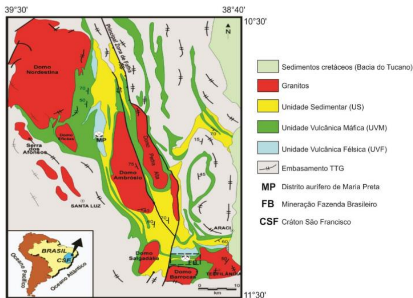
Figura 2: Mapa geológico simplificado do Greenstone Belt do Itapicuru (Rocha-Neto 1994).
