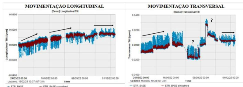
Figura 3. Gráficos de avaliação da estabilidade física da ETR da ECJ-CCR (linhas azuis – dados brutos e linhas vermelhas – dados suavizados) com indicativos de tendência (setas pretas) e intervalos sem possibilidade de definição de tendência (“?”).
