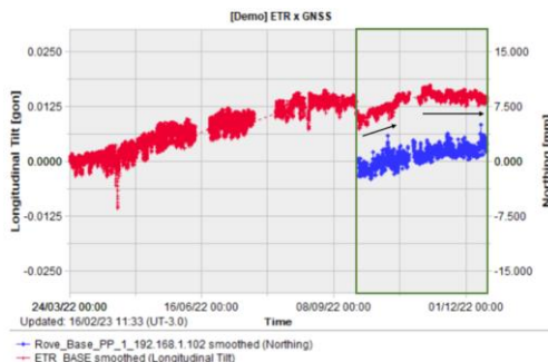
Figura 7. Gráficos de monitoramento da antena Rover do sistema GNSS da ECJ-CCR.
