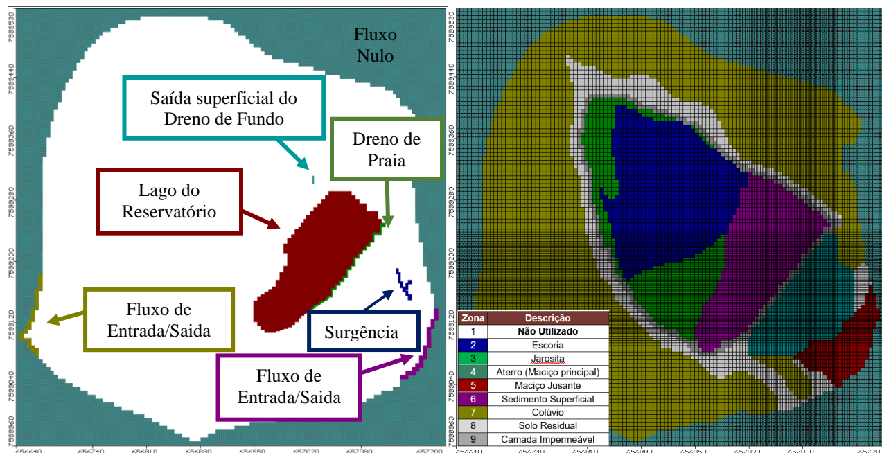
Figura 3. Condições de contorno imputadas ao modelo, com detalhe para as zonas de recarga superficiais (a direita), onde também é possível observar a malha utilizada com refino na área do maciço do barramento.
