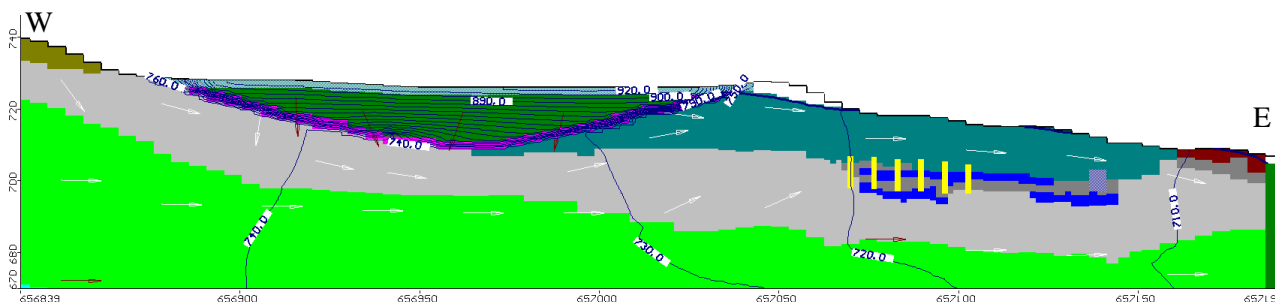
Figura 8. Equipotenciais e direções de Fluxo no Cenário 2 – Demais cores correspondem as zonas de condutividade hidráulica
