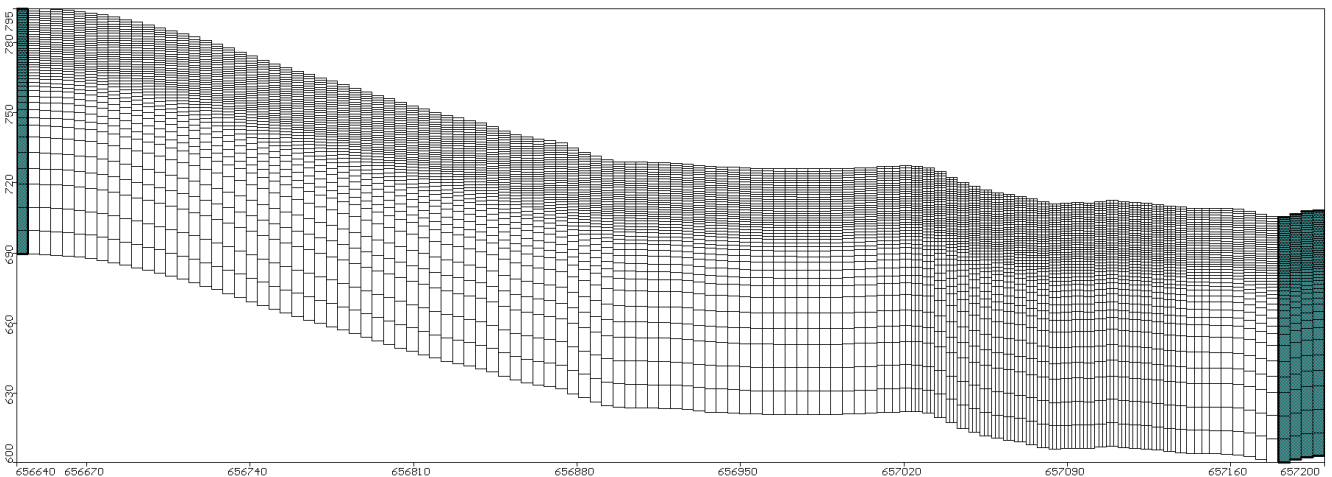
Figura 2 – Malha vertical do modelo numérico.
