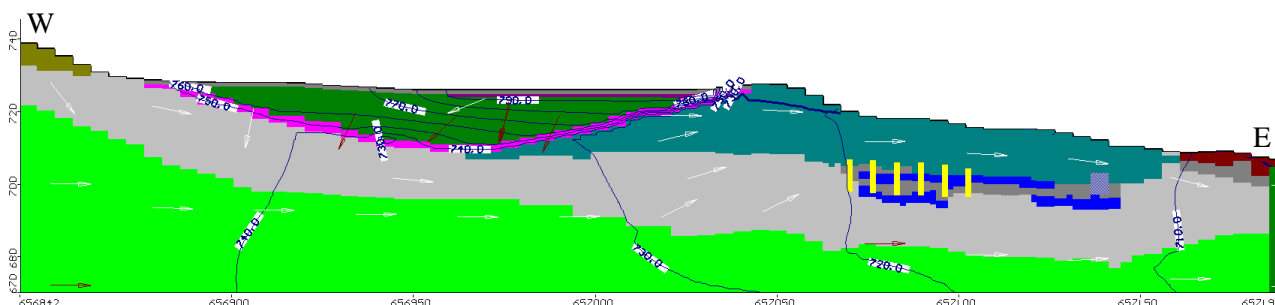
Figura 7. Equipotenciais e direções de Fluxo no Cenário 1 – Demais cores correspondem as zonas de condutividade hidráulica.
