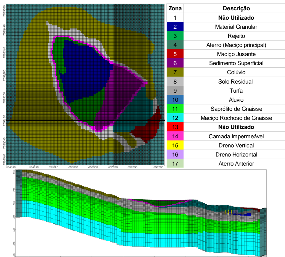
Figura 4. Unidades hidrogeológicas discretizadas no modelo em planta e seção.
