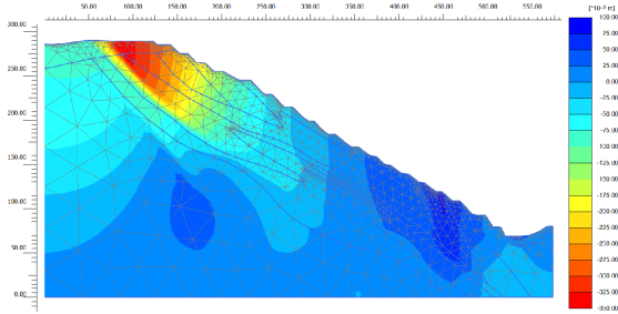
Figura 8: Deslocamentos no eixo vertical da seção B-B'.
