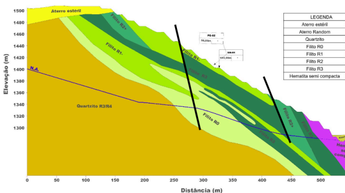
Figura 4: Seção transversal correspondente a da Seção B-B’.
