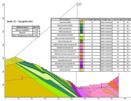
Figura 15: Análise de ruptura circular da seção C-C'.
