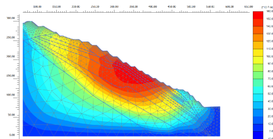
Figura 11: Deslocamentos no eixo horizontal da seção C-C'.
