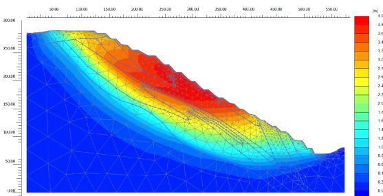
Figura 10: Deslocamentos no eixo horizontal da seção B-B'.
