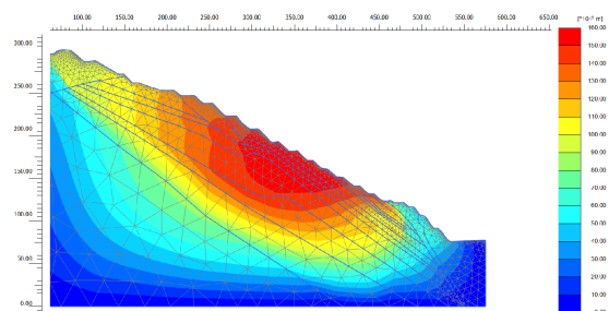
Figura 13: Deslocamentos total da seção C-C'.
