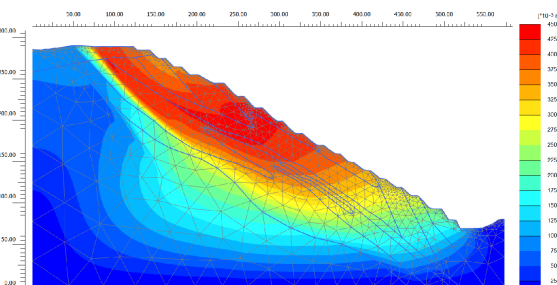
Figura 12: Deslocamentos total da seção B-B'.
