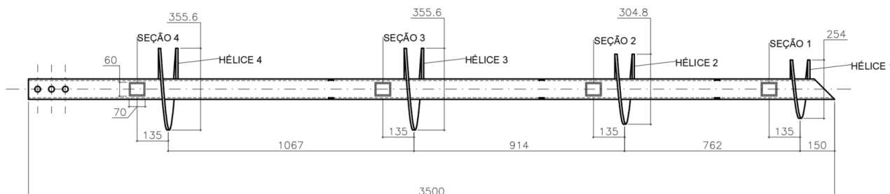
Figura 1. Detalhe da seção guia da estaca com 4 hélices (medidas em mm).
