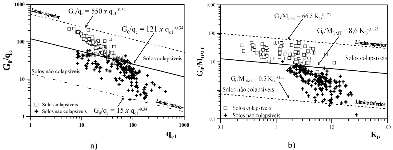
Figura 6. a) Limites superior e inferior que separam solos colapsíveis de solos não colapsíveis a partir da relação (a) G_0/q_c v q_{c1} (a) e (b) G_0/M_{DMT} vs K_D (adaptado de ROCHA et al., 2021, 2023).
