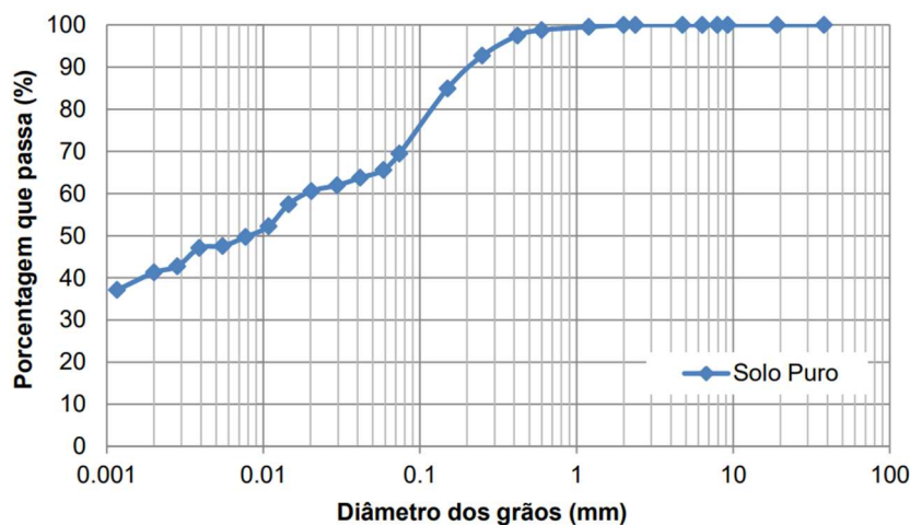
Figura 3. Análise granulométrica feita no solo sem adição de fibras.
