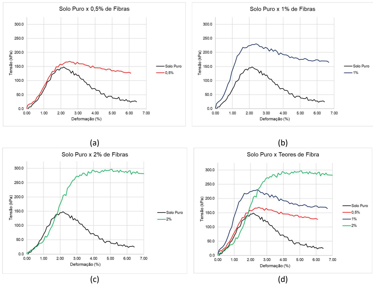
Figura 4. Curvas tensão-deformação para corpos de prova de solo puro e com fibras de resíduos têxteis: (a) 0,5% de fibra; (b) 1,0% de fibra; (c) 2,0% de fibra; (d) comparação entre todas as porcentagens de fibra.
