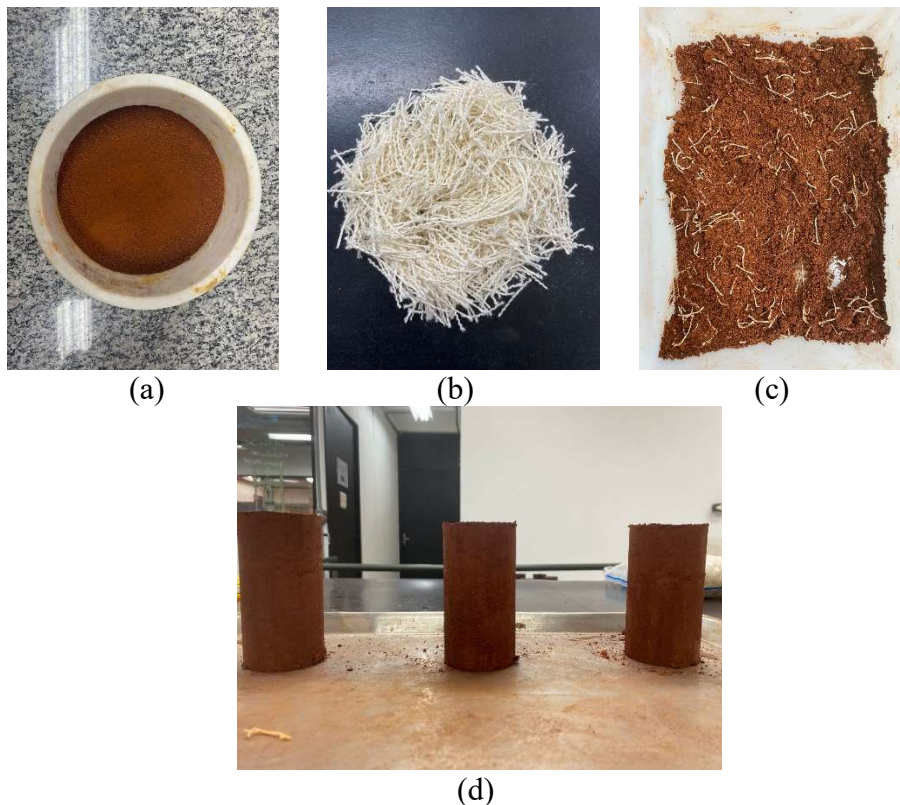
Figura 2. (a) Solo tropical laterítico argiloso. (b) Fibras de algodão obtidas a partir de resíduos têxteis. (c) Mistura solo-fibras. (d) Corpos de prova solo-fibras.
