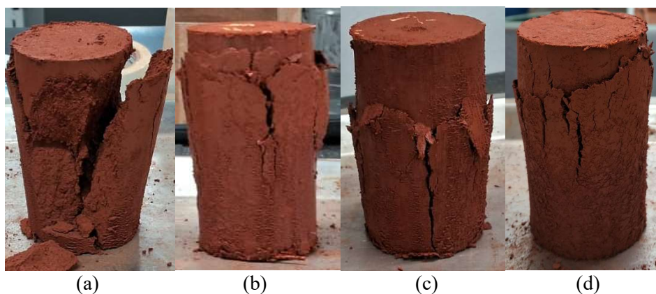
Figura 5. Formas de ruptura dos corpos de prova do: (a) solo natural sem reforço, (b) solo reforçado com 0,5% de fibra, (c) solo reforçado com 1,0% de fibra e (d) solo reforçado com 2,0% de fibra.
