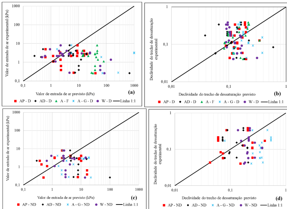
Figura 1. Previsão dos parâmetros da CCSA para solos naturais bimodais: a) valor de entrada de ar empregando granulometria com dispersão; b) declividade do trecho de dessaturação empregando granulometria com dispersão; c) valor de entrada de ar empregando granulometria sem dispersão; d) declividade do trecho de dessaturação empregando granulometria sem dispersão.
