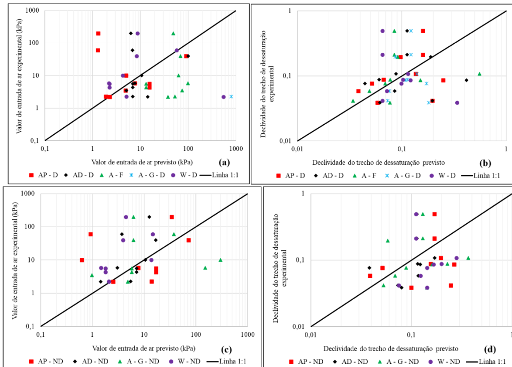
Figura 2. Previsão dos parâmetros da CCSA para solos compactados bimodais: a) valor de entrada de ar empregando granulometria com dispersão; b) declividade do trecho de dessaturação empregando granulometria com dispersão; c) valor de entrada de ar empregando granulometria sem dispersão; d) declividade do trecho de dessaturação empregando granulometria sem dispersão.
